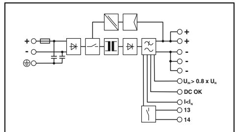
DC/DC-Wandler, schutzlackiert, 96 - 110 V DC / 24 V DC, 10 A
