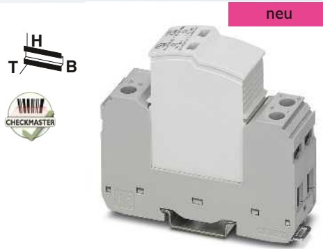
3-Leitersystem, DC+, DC-, PE für 380 V DC
