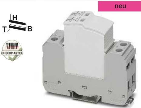
3-Leitersystem, DC+, DC-, PE für 220 V DC
