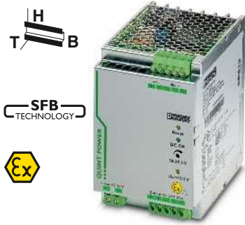
DC/DC-Wandler, schutzlackiert, 24 V DC / 24 V DC, 20 A
