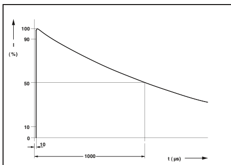
10/1000 Stoßstromimpuls nach IEEE C62.41.1
