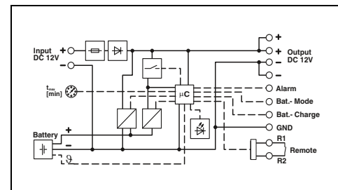
Unterbrechungsfreie Stromversorgung mit integriertem Batteriemodul, 12 V DC / 12 V DC, 4 A
