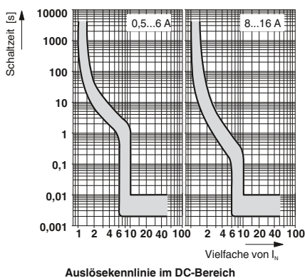
Auslösekennlinie im DC-Bereich
