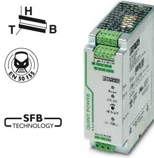
DC/DC-Wandler, schutzlackiert, 96 - 110 V DC / 24 V DC, 10 A
