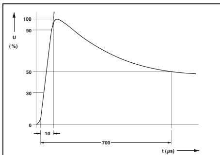
10/700 Stoßspannungsimpuls nach ITU-T K.44
