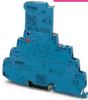
3-Leiter mit gemeinsamem Bezugspotenzial, eigensicher, steckbar
