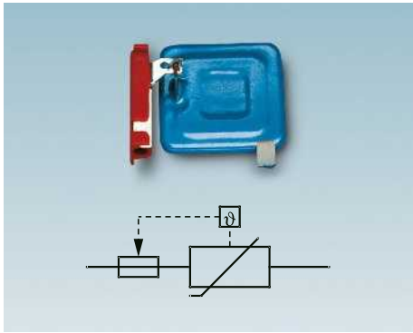
Blockvaristor mit thermischer Abtrennvorrichtung
