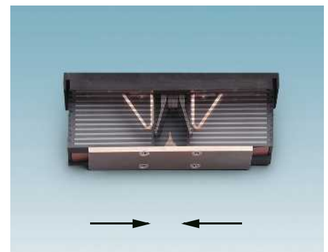
ARC-Funkenstrecke mit Löschblechen
