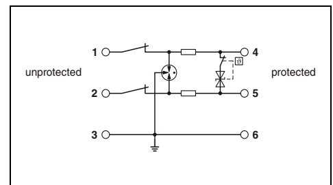
Doppelader (Loop), erdpotenzialfrei, Anschluss 3/6 direkt geerdet, mit Messertrennung, z. B. für 4 ... 20 mA Stromschleife
