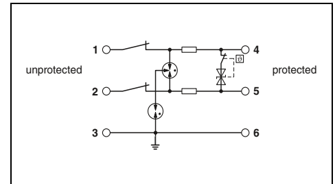
Doppelader (Loop), erdpotenzialfrei, eigensicher, steckbar, z. B. für 4 ... 20 mA Stromschleife
