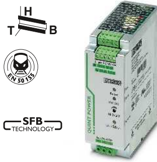
DC/DC-Wandler, schutzlackiert, 60 - 72 V DC / 24 V DC, 10 A
