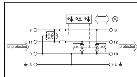
2-Leiter mit gemeinsamem Bezugspotenzial, Anschluss 9/10 direkt geerdet, z. B. für Binärsignale
