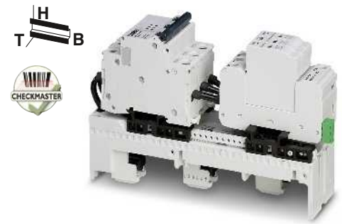
4-Leitersystem, L1, L2, L3, PEN für 60-mm-Systemtechnik
