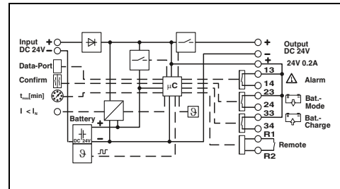
Unterbrechungsfreie Stromversorgung mit integriertem Energiespeicher, 24 V DC / 24 V DC, 10 A, 3.4 Ah
