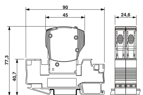
Abbildung zeigt das Kompletmodul, bestehend aus Basiselement und Stecker
