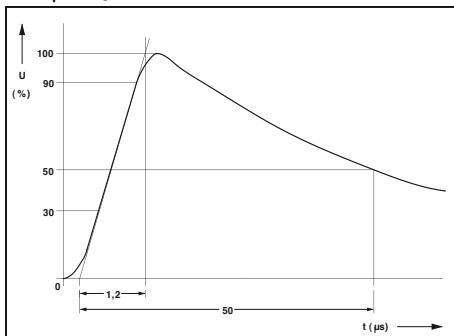
1,2/50 Stoßspannungsimpuls nach IEC 60060-1
