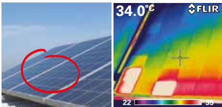
Defekte in Photovoltaik-Zellen lassen sich im Infrarotbild erkennen.
