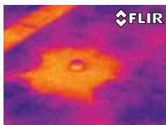
Das Thermografiebild zeigt Wasserlecks im Dach.
