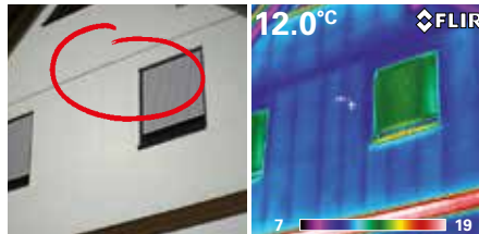
Eine fehlende Dämmung wird in der Wand erkannt. Zusätzlich wird die Ständerkonstruktion sichtbar.
