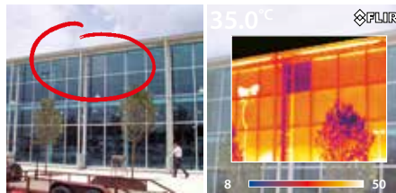
Die Thermografieinspektion deckt ein falsch eingebautes Fenster auf.
