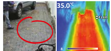
Fernwärmeleitung, aber nur ein Teil der Anlage funktioniert ordnungsgemäß.
